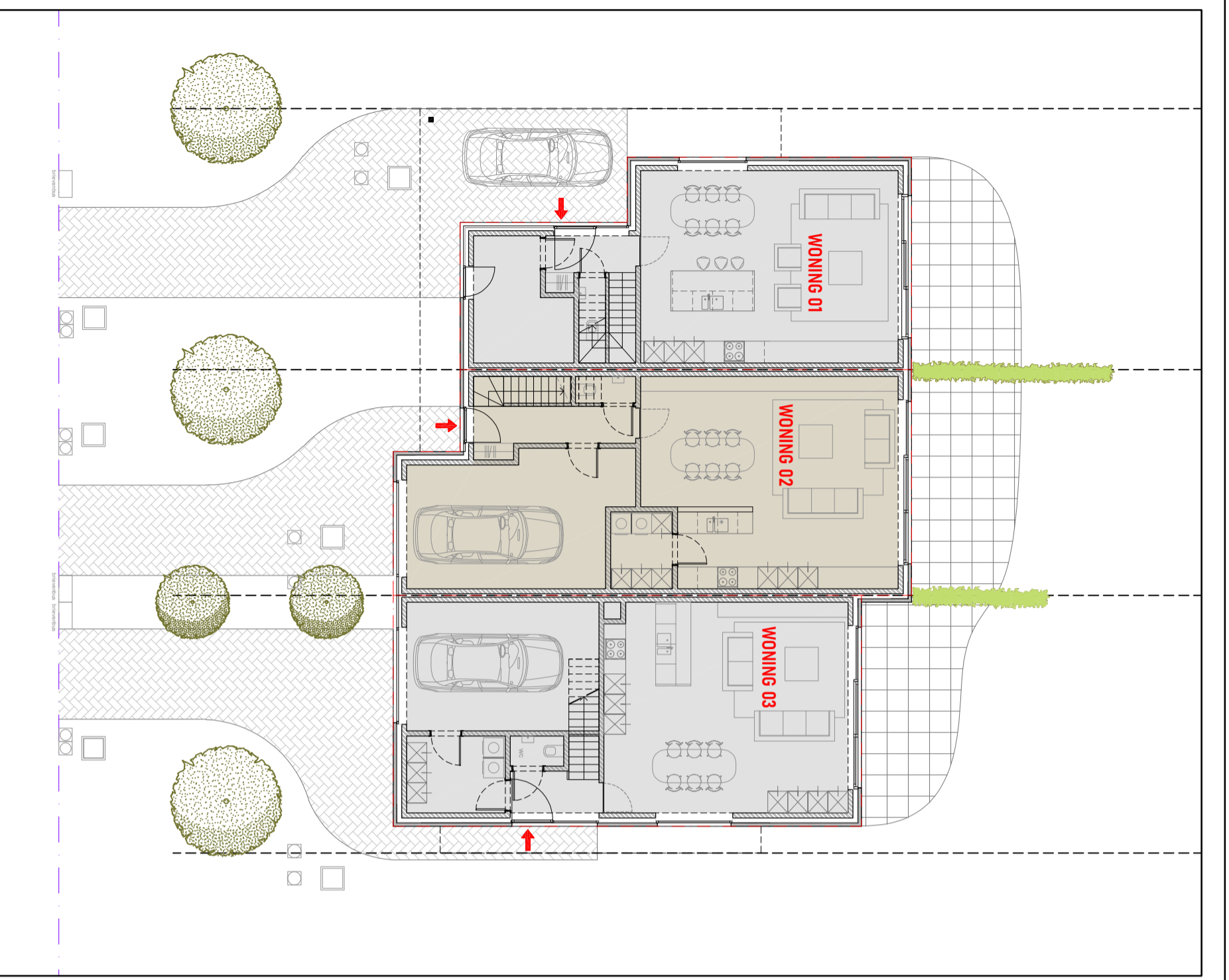
WONINGEN 1, 2 EN 3 - GELIJKVLOERS schaal 1:150
