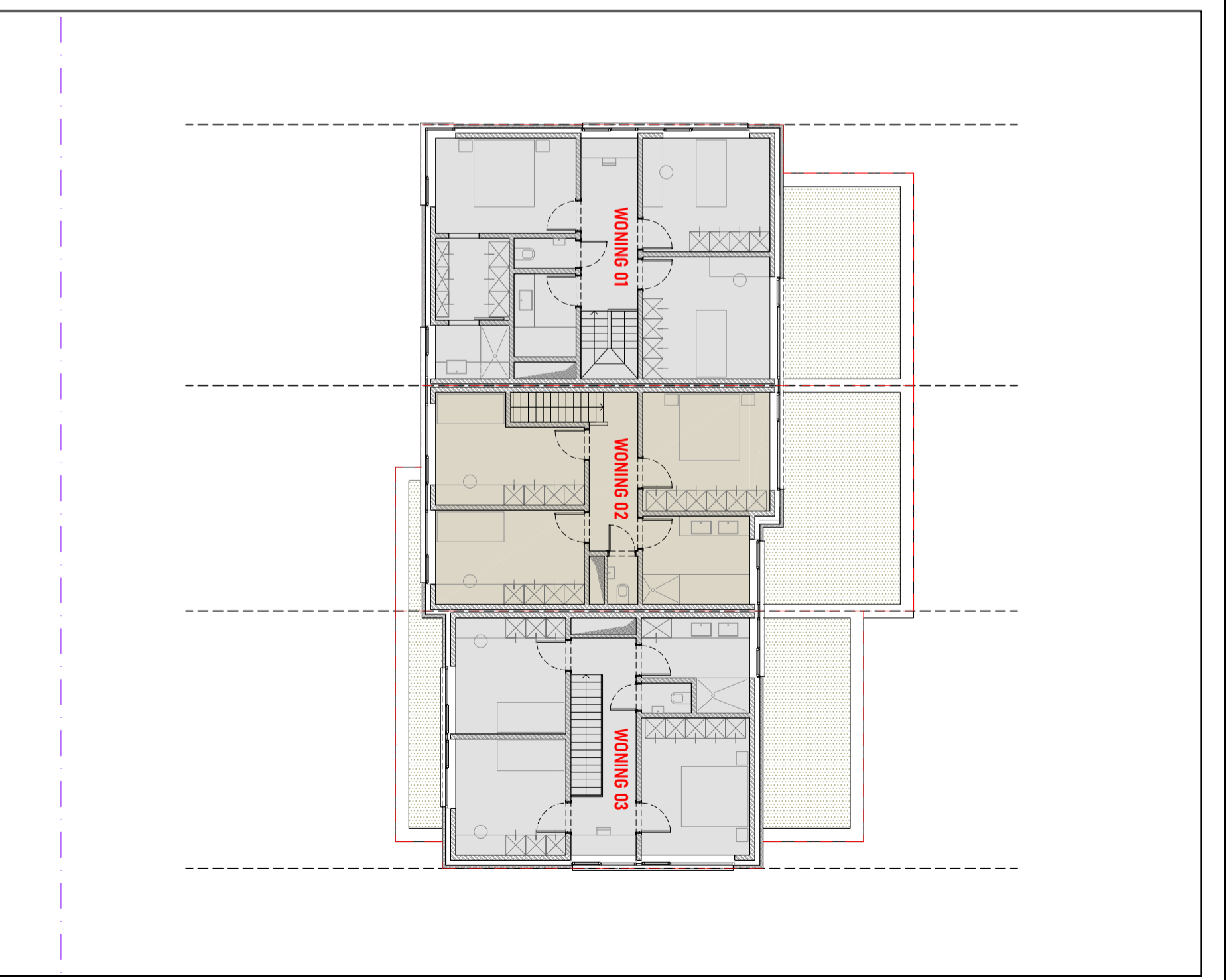
WONINGEN 1, 2 EN 3 - VERDIEPING 1 schaal 1:150
