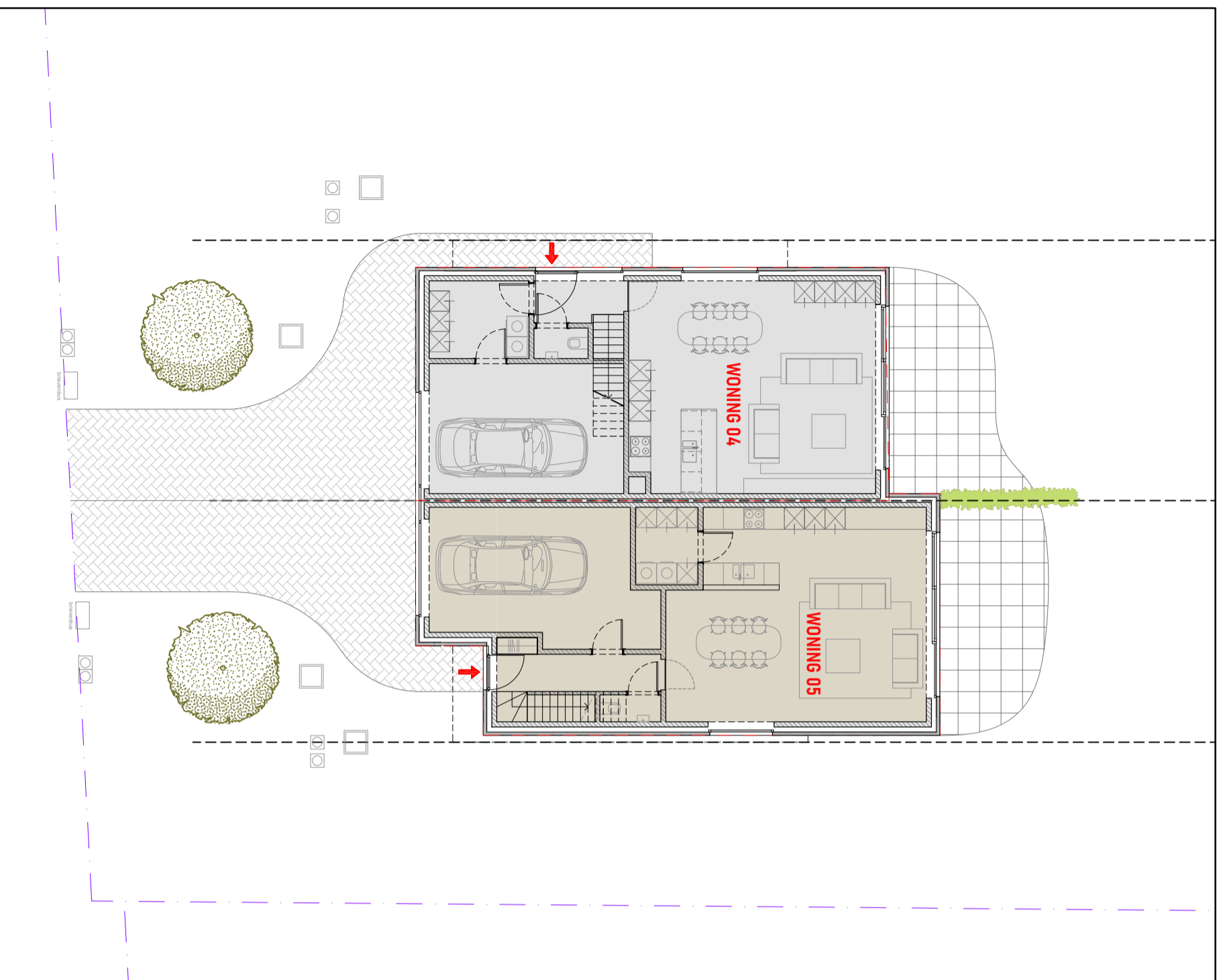
WONINGEN 4 EN 5 - GELIJKVLOERS schaal 1:150
