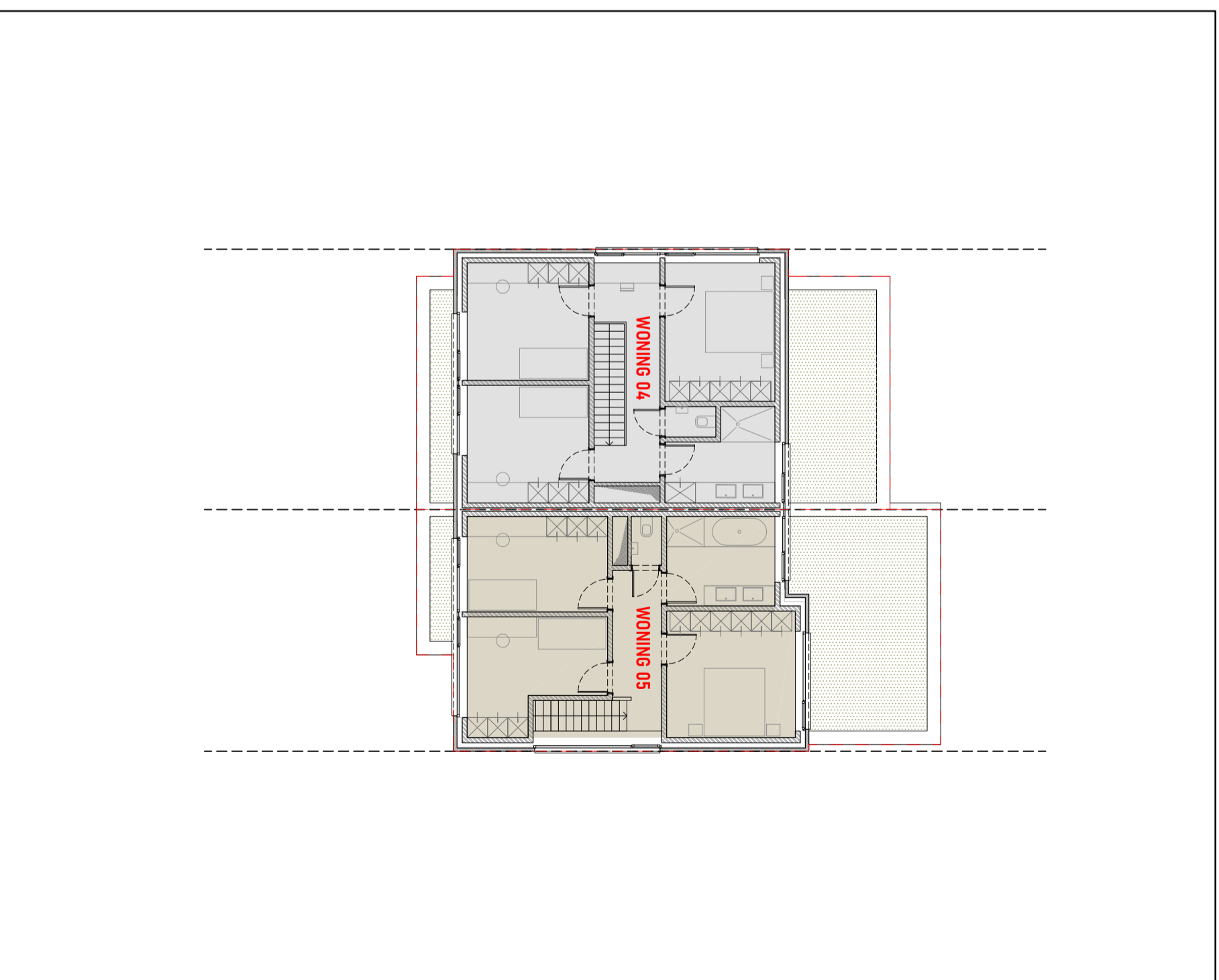
WONINGEN 4 EN 5 - VERDIEPING 1 schaal 1:150
